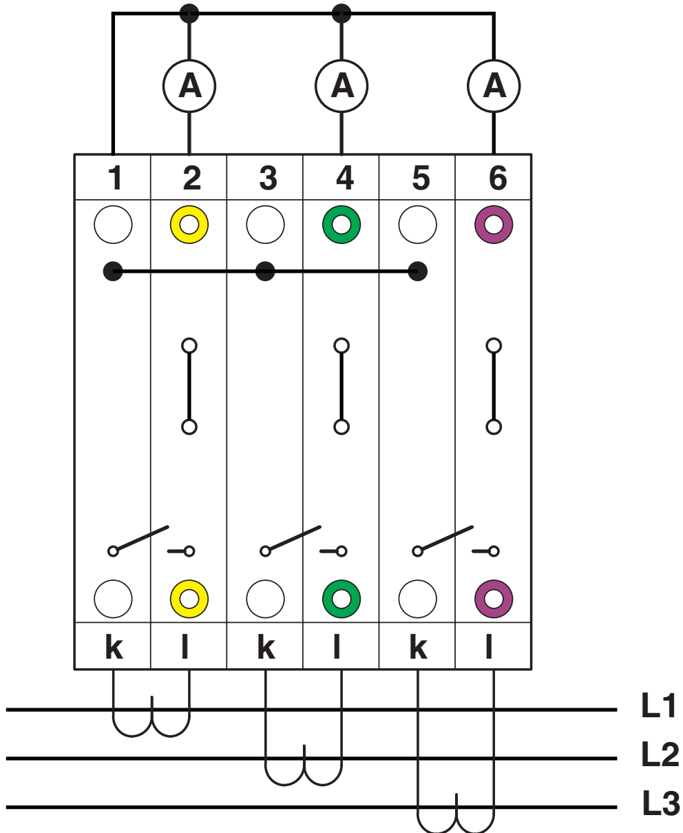
Tilkoblingstegning
