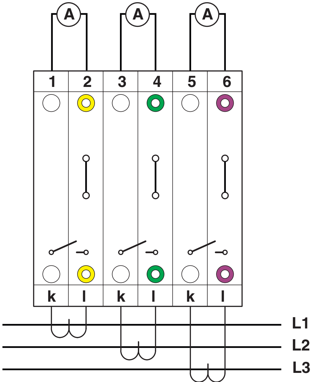
Tilkoblingstegning
