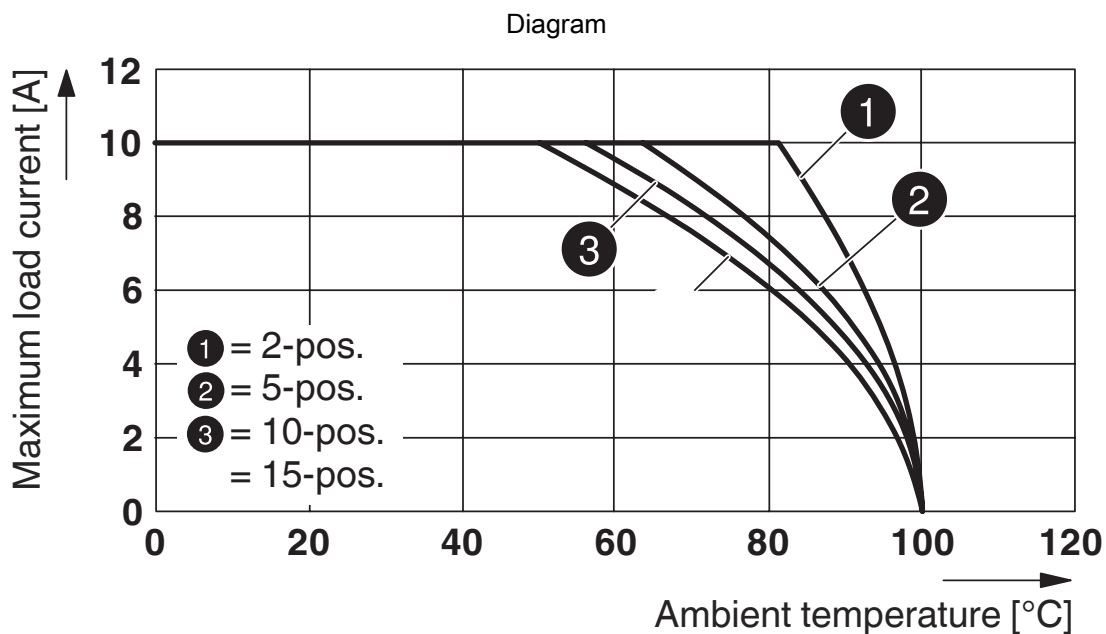
Deratingkurve for ST 2,5-4L/1P, ST 2,5-4L/2P og for alle stikkervarianter SP...
