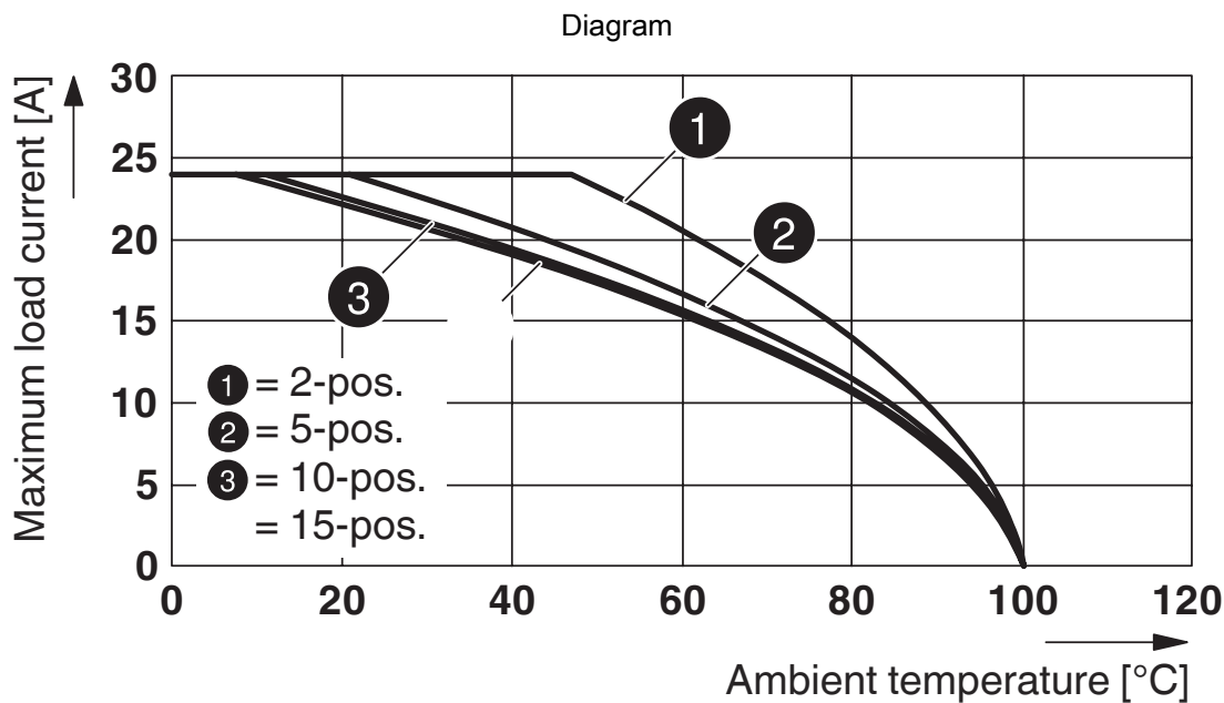
Deratingkurve for ST 2,5/ 1P, ST 2,5/ 2P, ST 2,5-TWIN/ 1P og for alle stikkervarianter SP...
