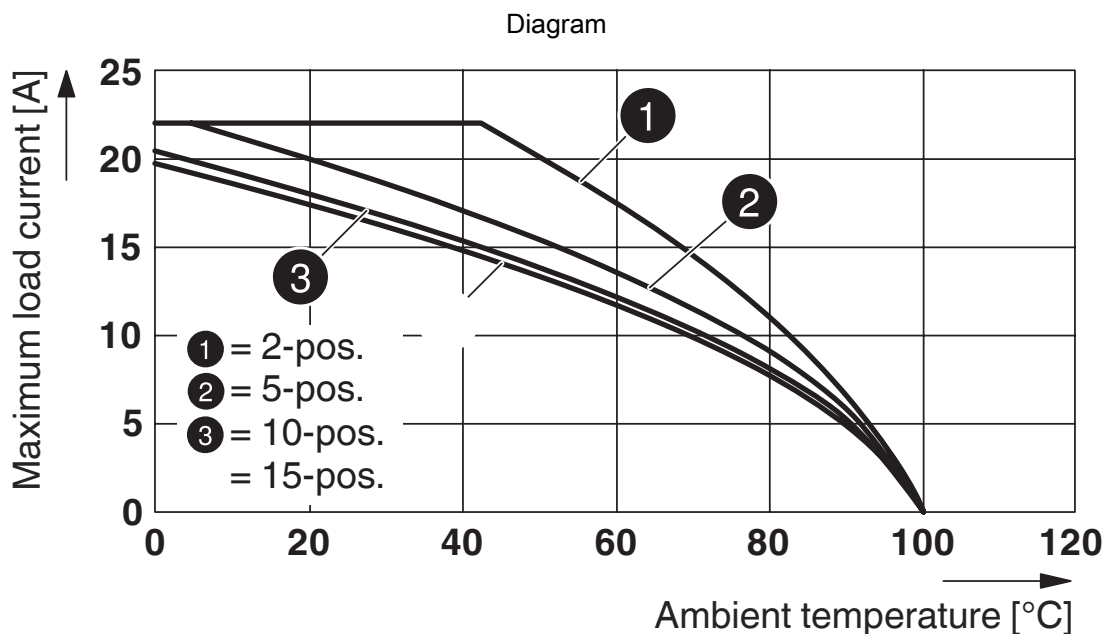
Deratingkurve for STTB 2,5/ 2P, STTB 2,5/ 2P-PV og for alle stikkervarianter SP...
