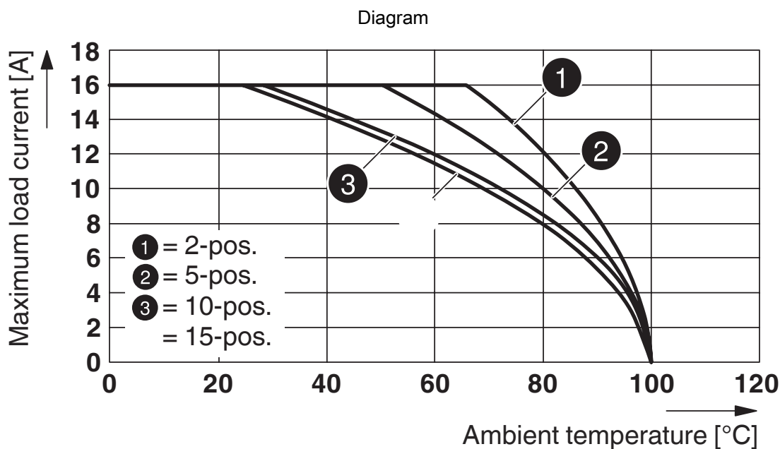
Deratingkurve for ST 2,5-TWIN-MT/1P, ST 2,5-TWIN-TG/1P og for alle stikkervarianter SP...
