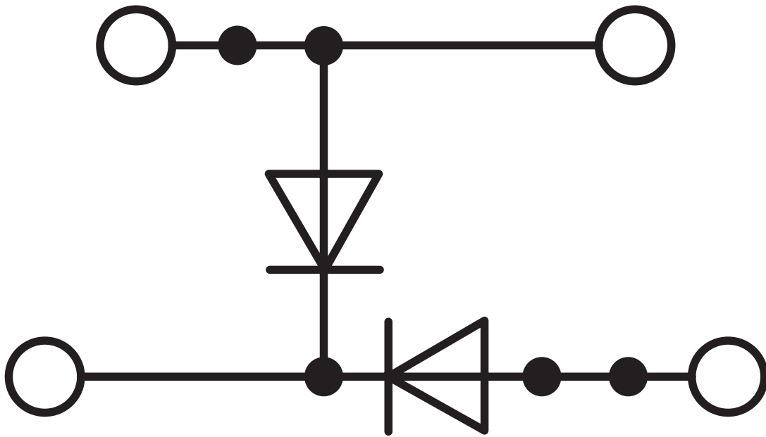
Koblingsskjema
