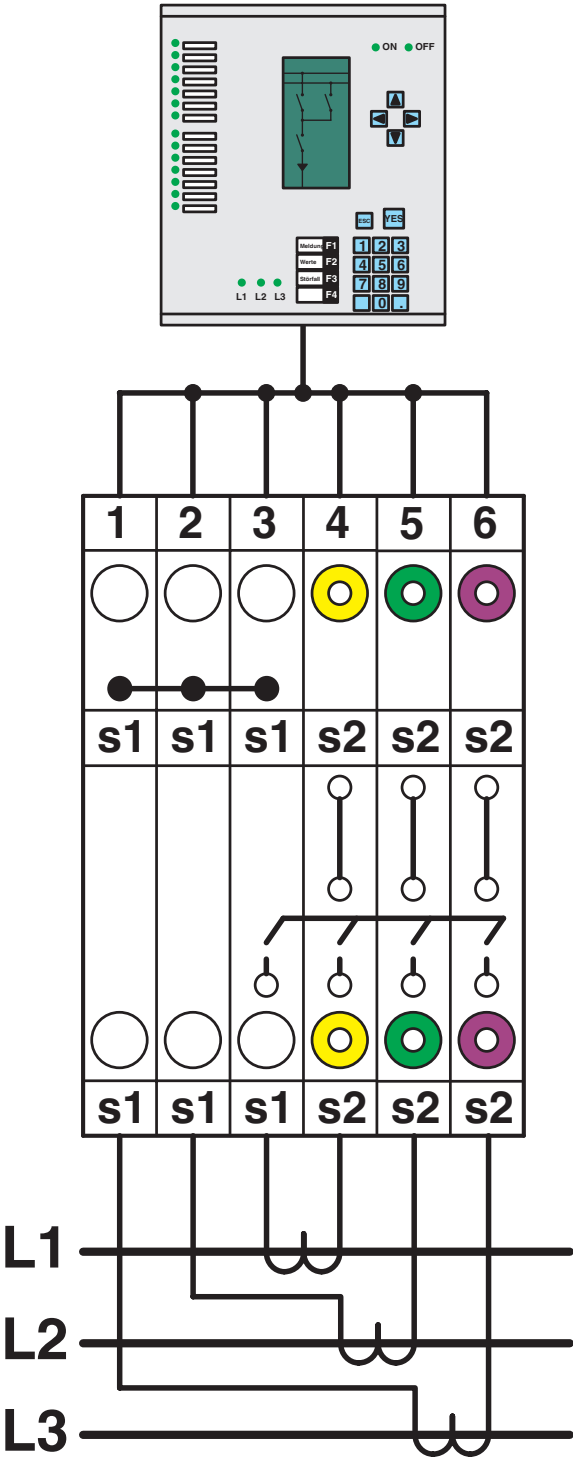
Skjemategning
