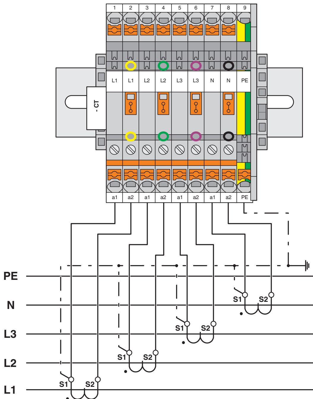
Koblingsskjema
