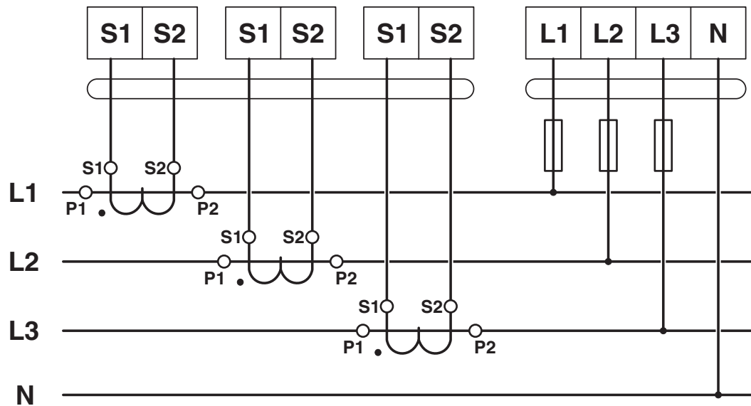
Koblingsskjema
