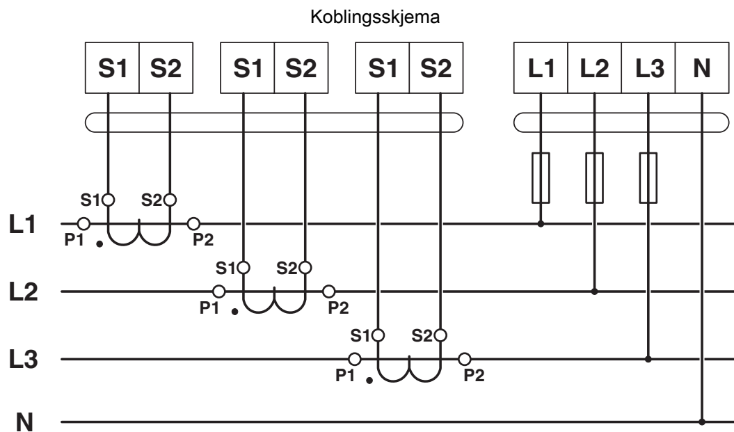
Koblingsskjema
