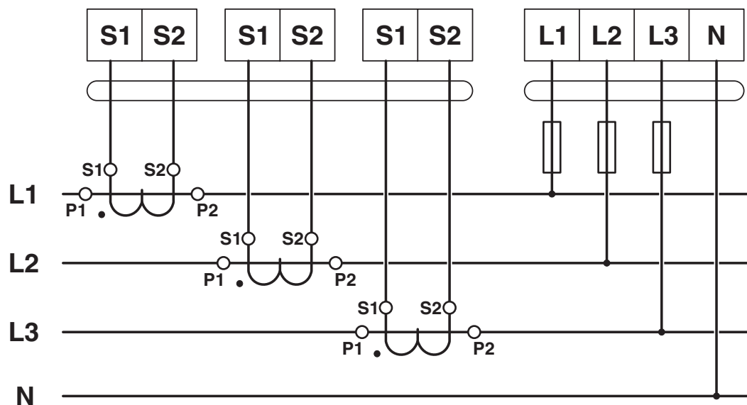
Koblingsskjema
