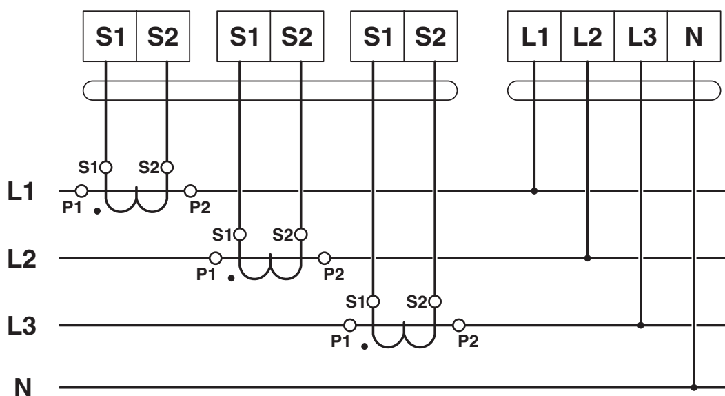
Koblingsskjema
