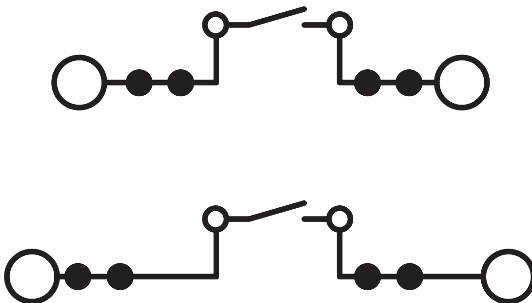
Koblingsskjema
