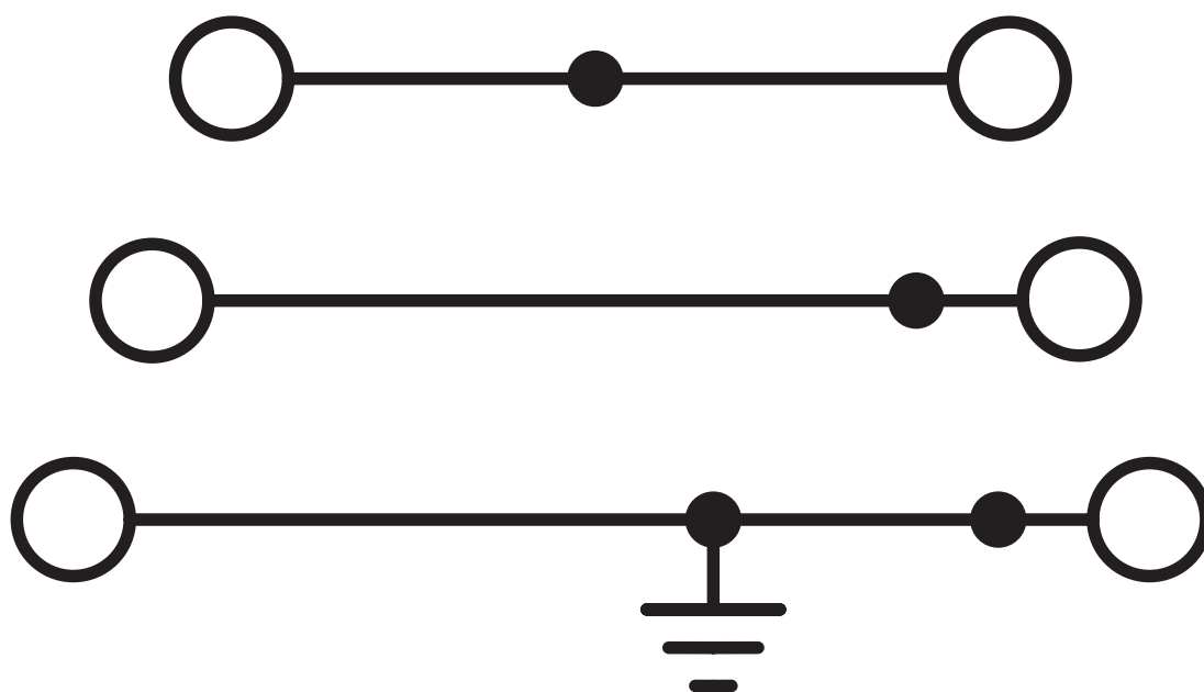
Koblingsskjema
