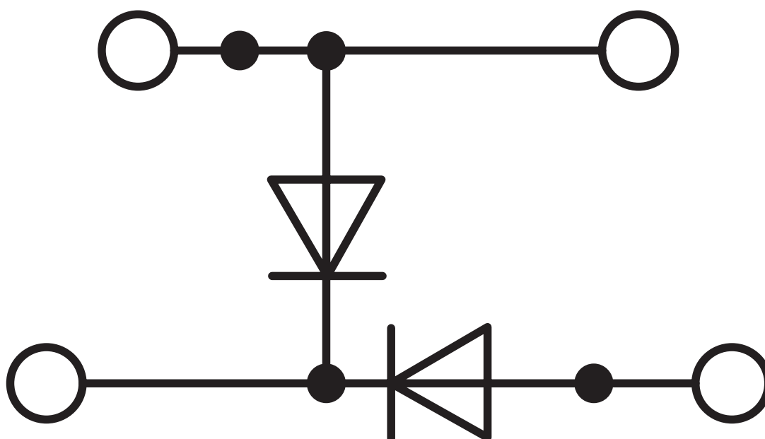
Koblingsskjema
