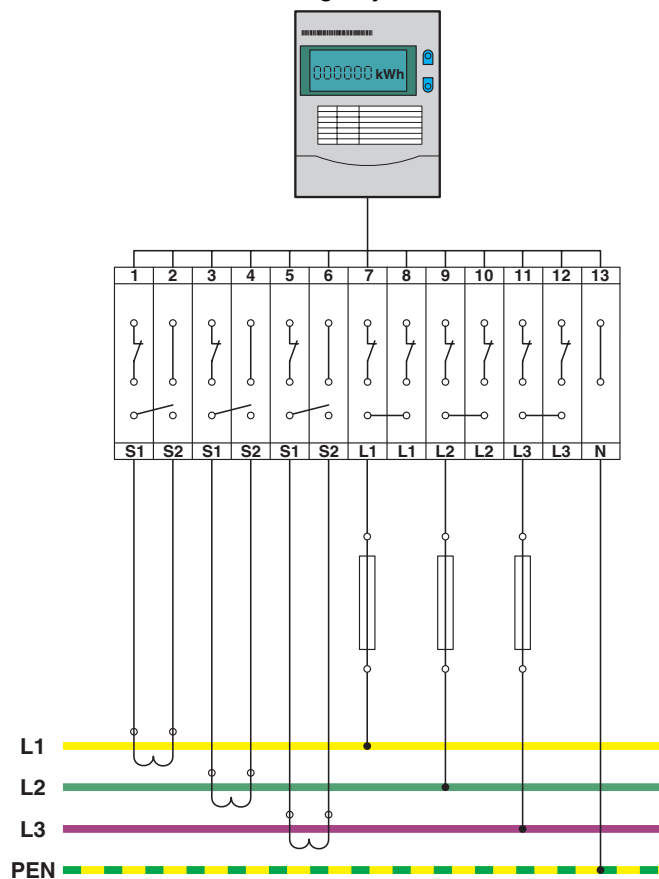
Koblingsskjema
