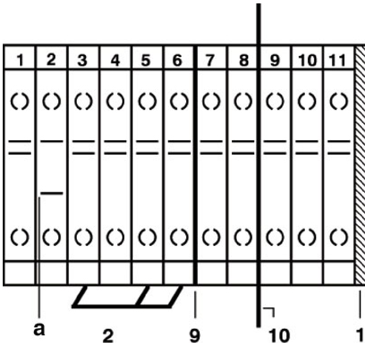
Koblingsskjema
