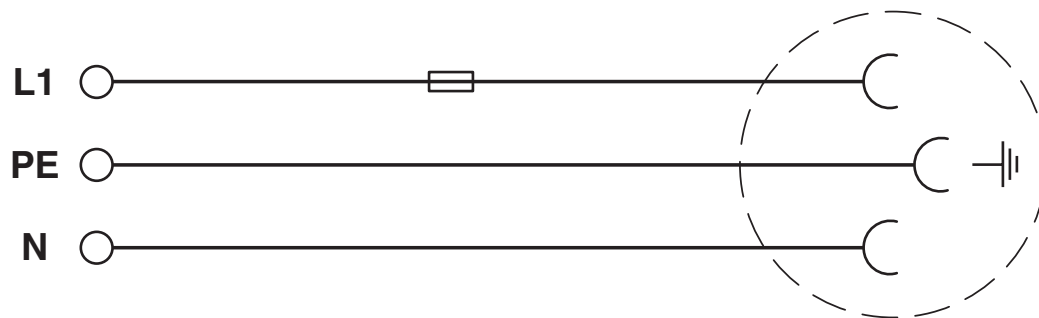
Koblingsskjema
