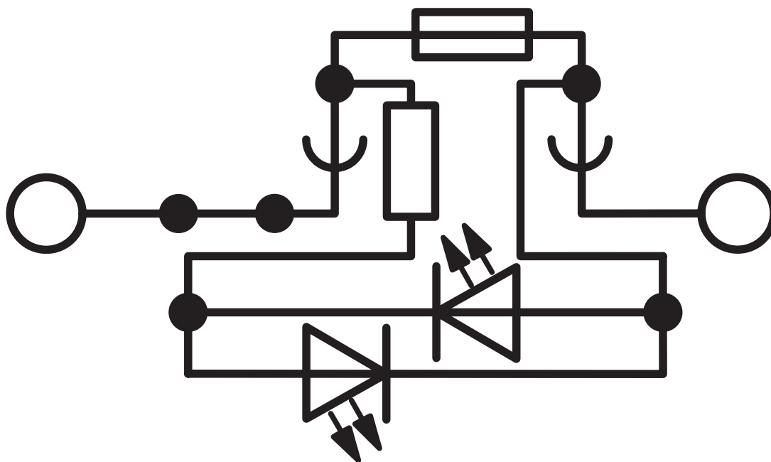
Koblingsskjema
