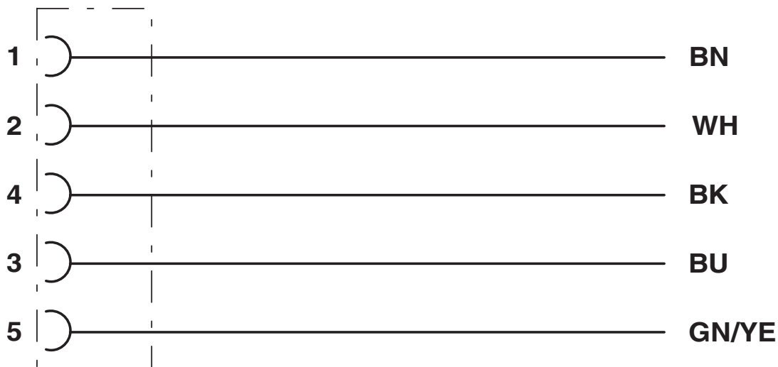
Koblingsskjema
