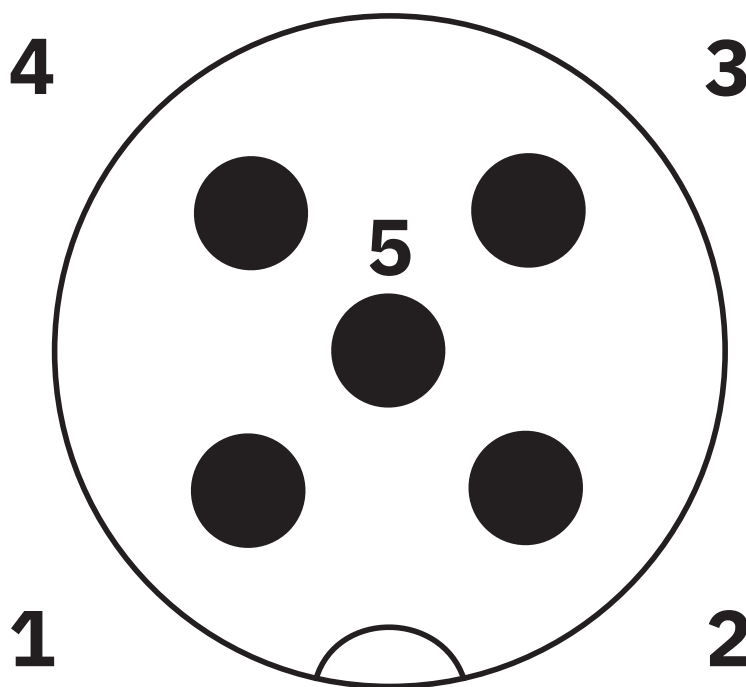
Skjemategning
