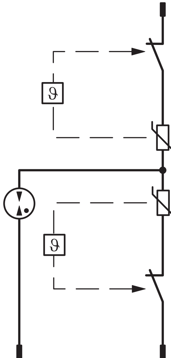
Koblingsskjema
