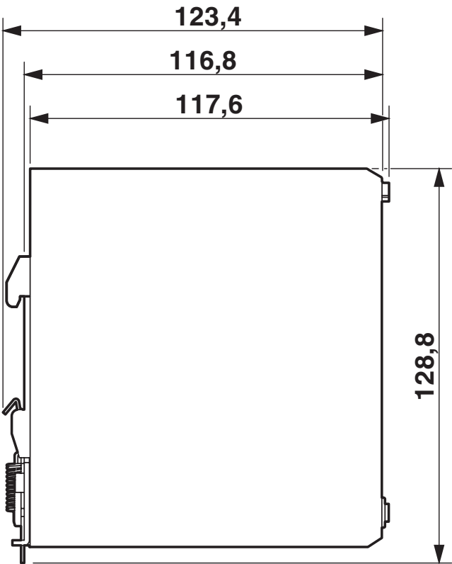
Målskisse
