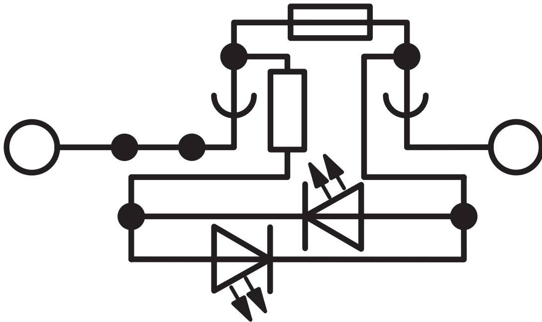
Koblingsskjema
