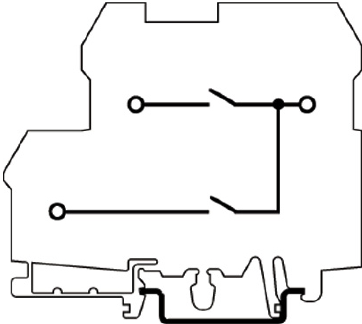
Koblingsskjema
