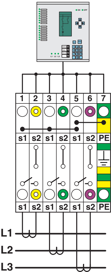
Skjemategning
