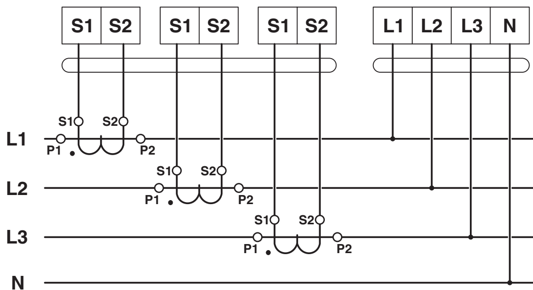
Koblingsskjema
