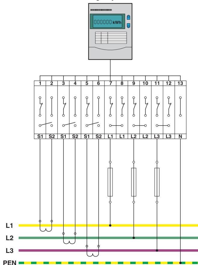
Koblingsskjema
