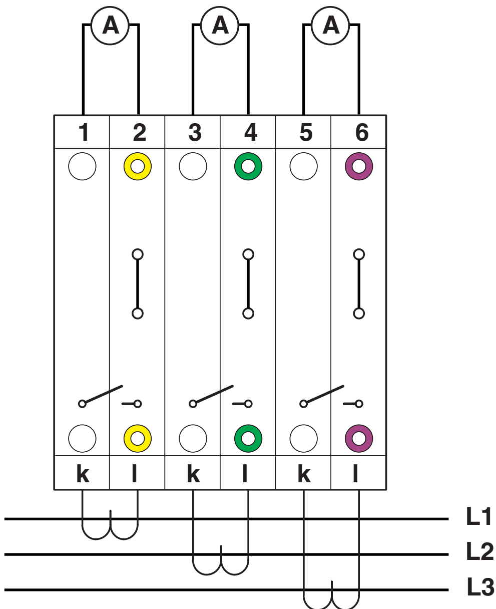
Tilkoblingstegning
