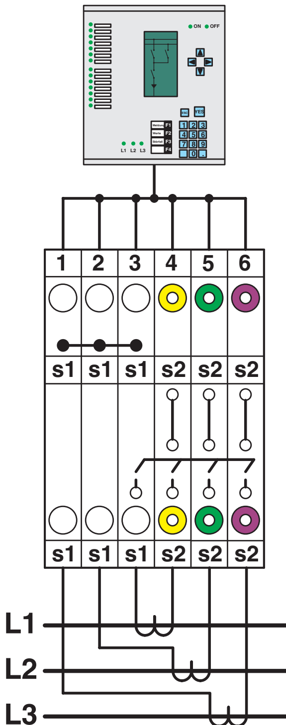
Skjemategning
