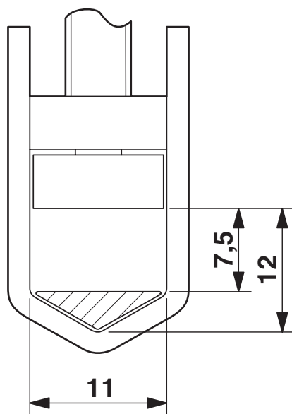
Målskisse
