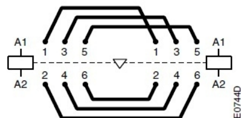
BEM... connections
