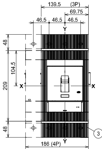
Front for copper cables - FC Cu or for copper/aluminium cables - FC CuAl
