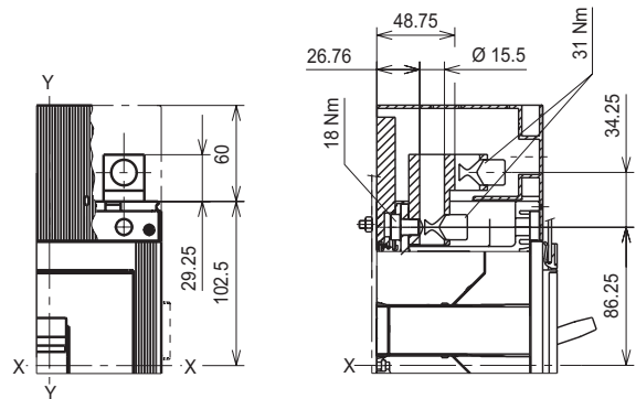
Front for copper/aluminium cables - FC CuAl 300 mm 2
