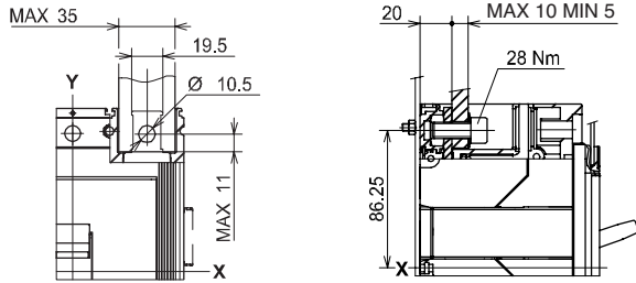
Front for copper/aluminium cables - FC CuAl
