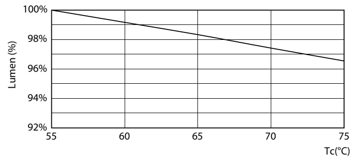
Lumen Maintenance Diagram - CorePro LEDtube UN 1500mm UO 23W865 T8
