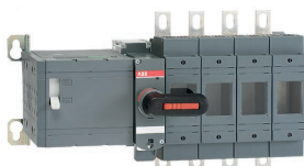
OSM200D4N2M230C
