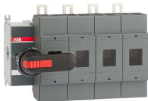
OS400J04F
