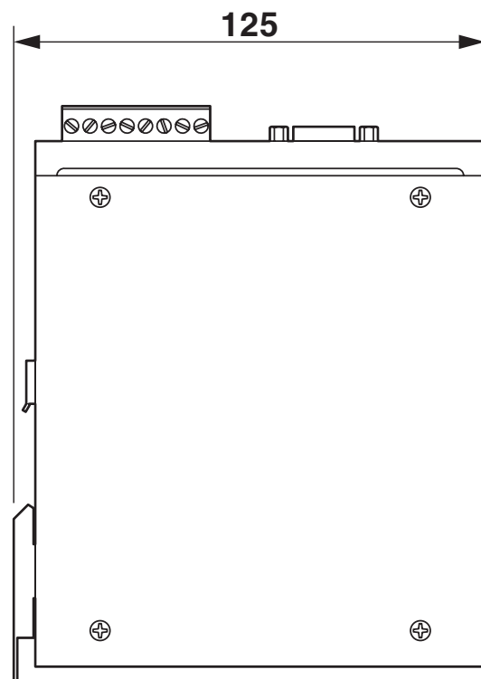
Målskisse
