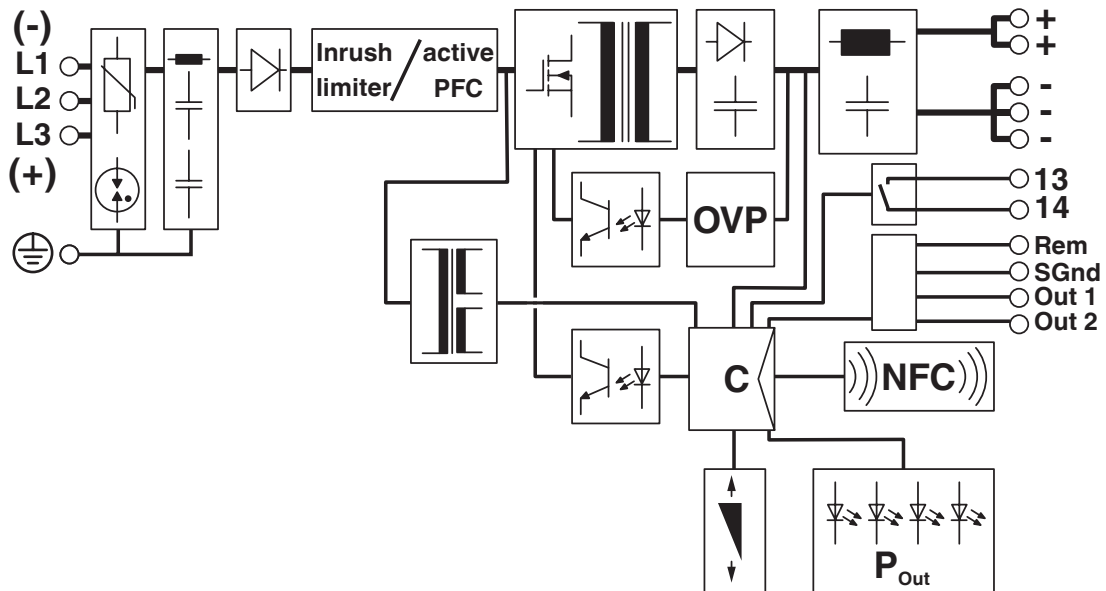
Blokkskjema
