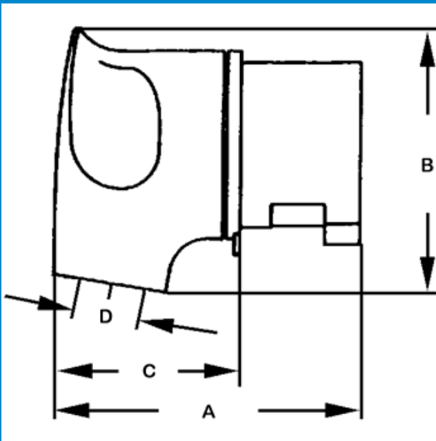
Målskisse
