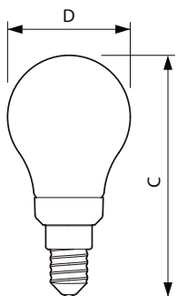
Candle P45 230V 5-35W 400lm 2500K E14 D
