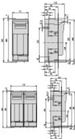
2x XNH32-1-A...
