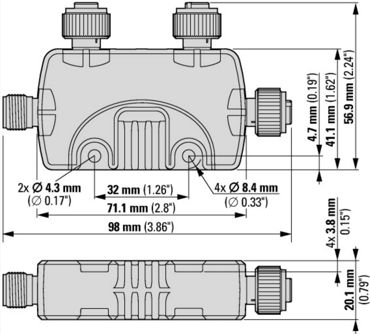
SmartWire-DT I/O modules (IP67) EU2E-SWD-....
