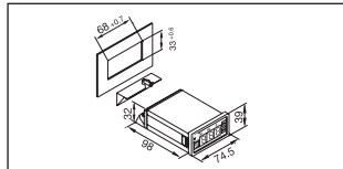
Abb. 1: Gerätemontage Fig. 1: Assembly Fig. 1: Montage de l'appareil Afb. 1: Apparatmontage Bild 1: Apparatmontage Fig. 1: Montaggio dell'apparecchio Imagen 1: Montaje del aparato 図 1: 組立
