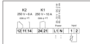
Abb. 3: Anschlussschema Fig. 3: Connection diagram Fig. 3: Schema de connexion Afb. 3: Aanslutningschema Bild 3: Anslutningsschema Fig. 3: Schema d'alimentazione Imagen 3: Esquema de conexión 図 3: 結線図
