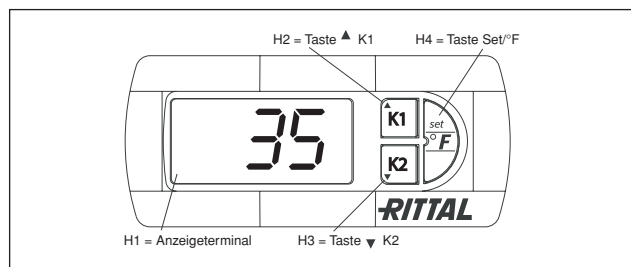
Abb. 6.1 Elektronische Regelung
