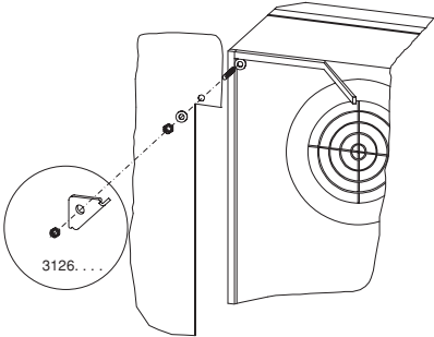
Abb. 3.2 Gerätemontage Fig. 3.2 Mounting Fig. 3.2 Montage de l'appareil Afb. 3.2 Apparaatmontage Bild 3.2 Aggregatmontage Fig. 3.2 Montaggio dell'apparecchio Fig. 3.2 Montaje del aparato
