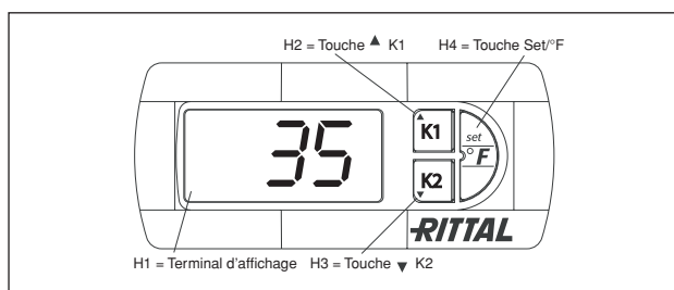
Fig. 6.1 Régulation électronique
