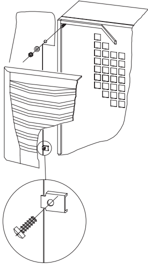
Einbau Internal mounting Montage encastré Inbouw Inbyggnad Incassato Montaje interior
