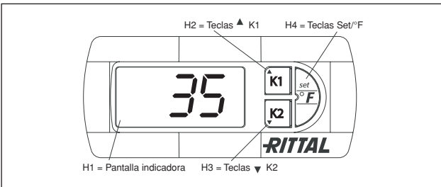
Figura 6.1 Regulación electrónica
