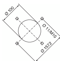
Montageausschnitt
