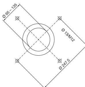
Montageausschnitt
