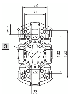
Ansicht B
