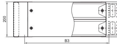
Sokkel 200 mm høy
