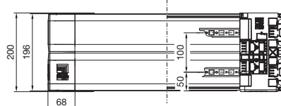
Flex-Block 200 mm høy
