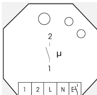
Funksjonsvelgere (Fabrikkinnstilling)
