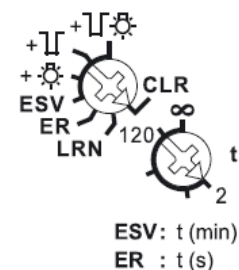
Funksjonsvelgere (Fabrikkinnstilling)
