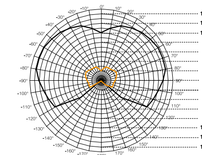
Dekningsområde L 400S · L 410S Monteringshøyde 2,8 m Svart = tangential gangretning Oransje = radial gangretning
