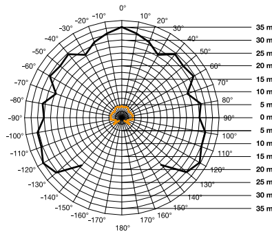
Dekningsområde sensIQ KNX Monteringshøyde 1,8 m Svart – tangential gangretning Oransje – radial gangretning
