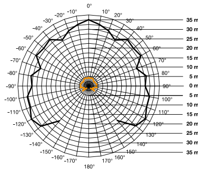
Dekningsområde sensIQ S Monteringshøyde 1,8 m Svart – tangential gangretning Oransje – radial gangretning
