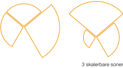
Dekningsområde sensIQ S Monteringshøyde 1,8 m Svart – tangential gangretning Oransje – radial gangretning
