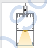
Schnell-Befestigungssystem quick attachment system
