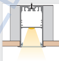
Montage mit Einbaubügel für Hohlraumdecken mounting with installation bracket for suspended ceilings
