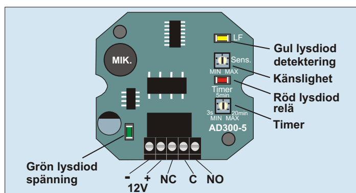
Kretskort med anslutningsplint
