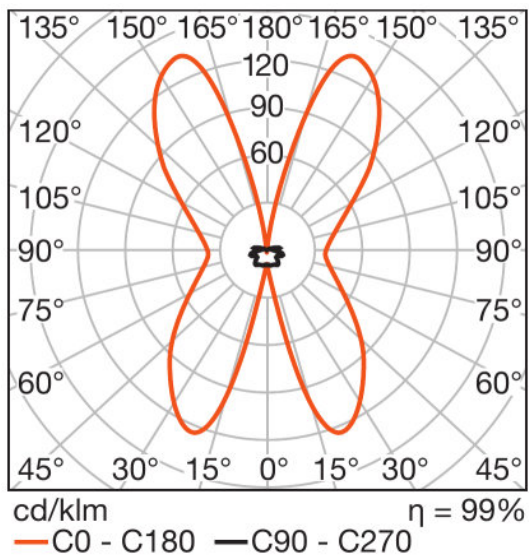
LDC typ luminance
