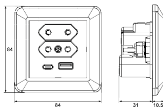
Målskisse
