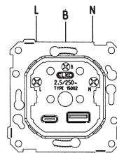
Koblingsskjema
