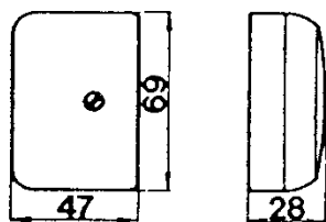
Målskisse
