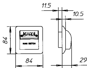
Målskisse
