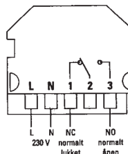
Koblingsskjema
