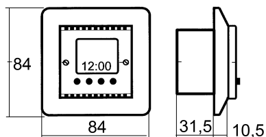
Målskisse
