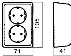
Målskisse
