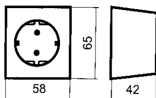
Målskisse
