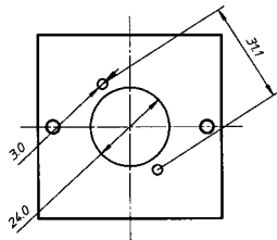
Målskisse
